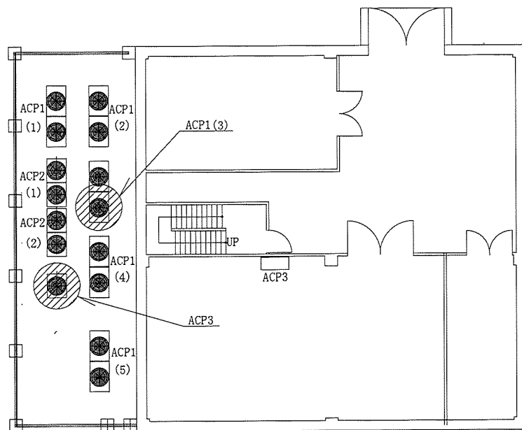
#77平面図(1F)
