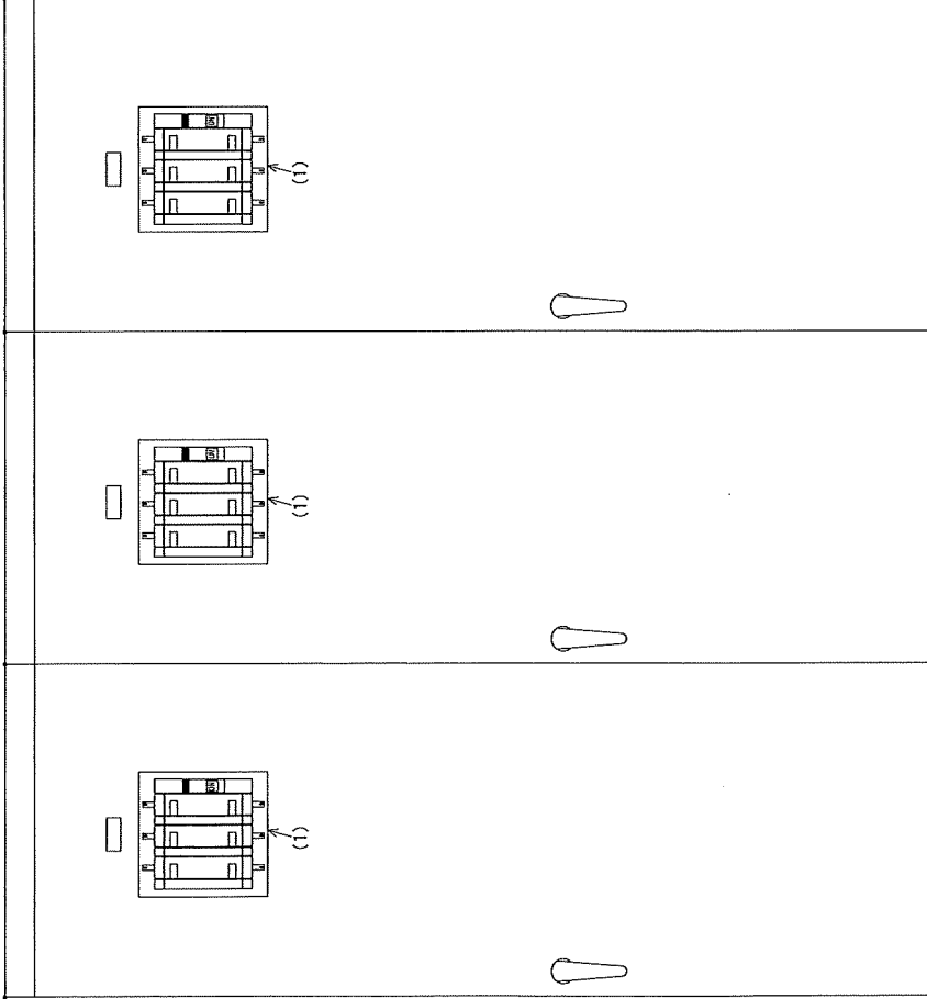
動力配電盤P-1(No.1)撤去 (正面図) 動力配電盤P-1(No.2)撤去 (正面図) 動力配電盤P-1(No.3)撤去 (正面図)
