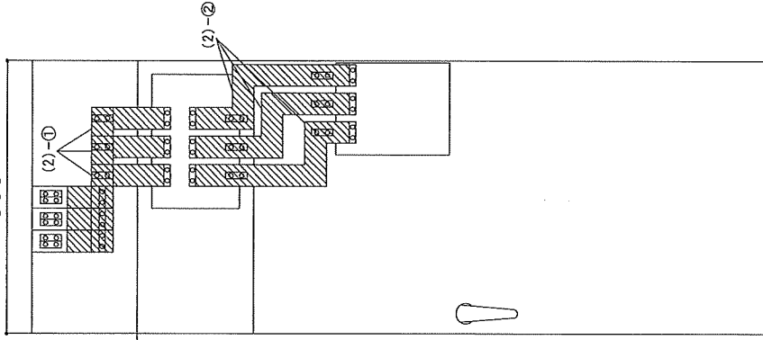
NONTECH-2盤撤去（裏面図）
