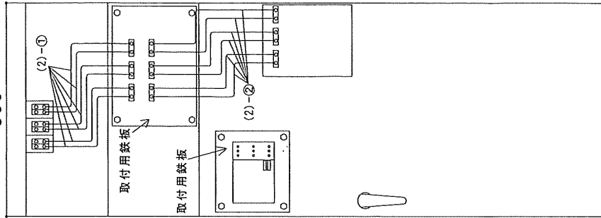
TECH-4盤設置（裏面図）
