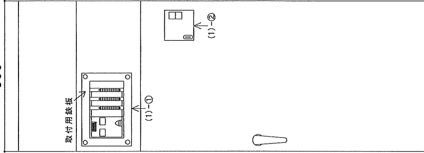
TECH-4盤設置（正面図）
