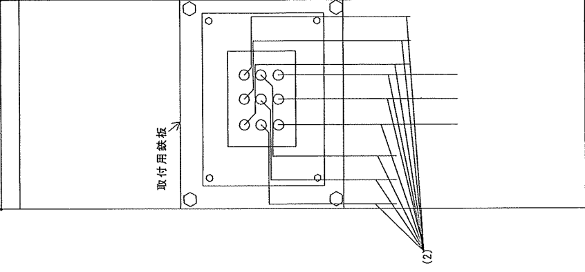
配電盤設置 (裏面図)
