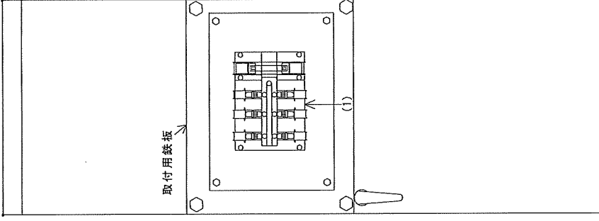
配電盤設置 (正面図)
