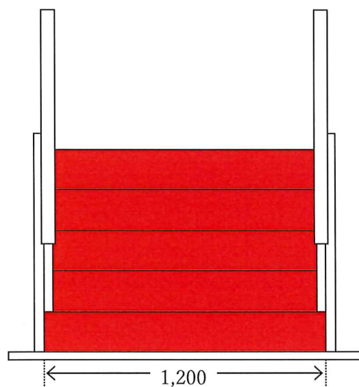
<手すり付き階段正面図>
