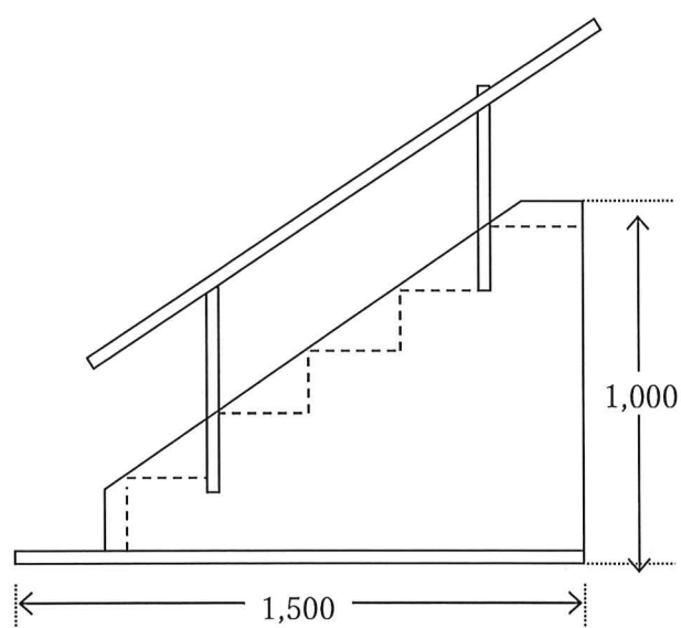
<手すり付き階段側面図>
