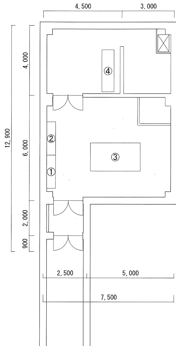
A局舎電源室平面図 S-1/150
