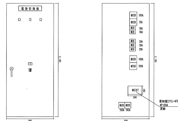
⑦ 電源切換盤姿図 N/S
