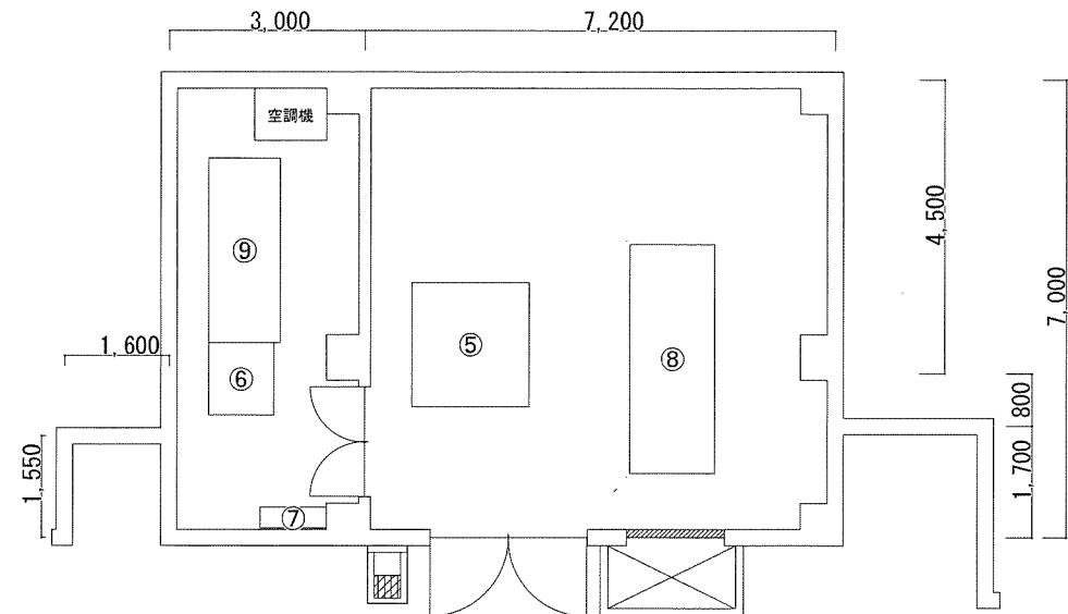
B局舎電源室平面図 S-1/200
