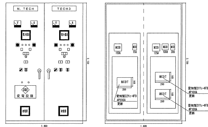
⑤ 電源切換盤姿図 N/S
