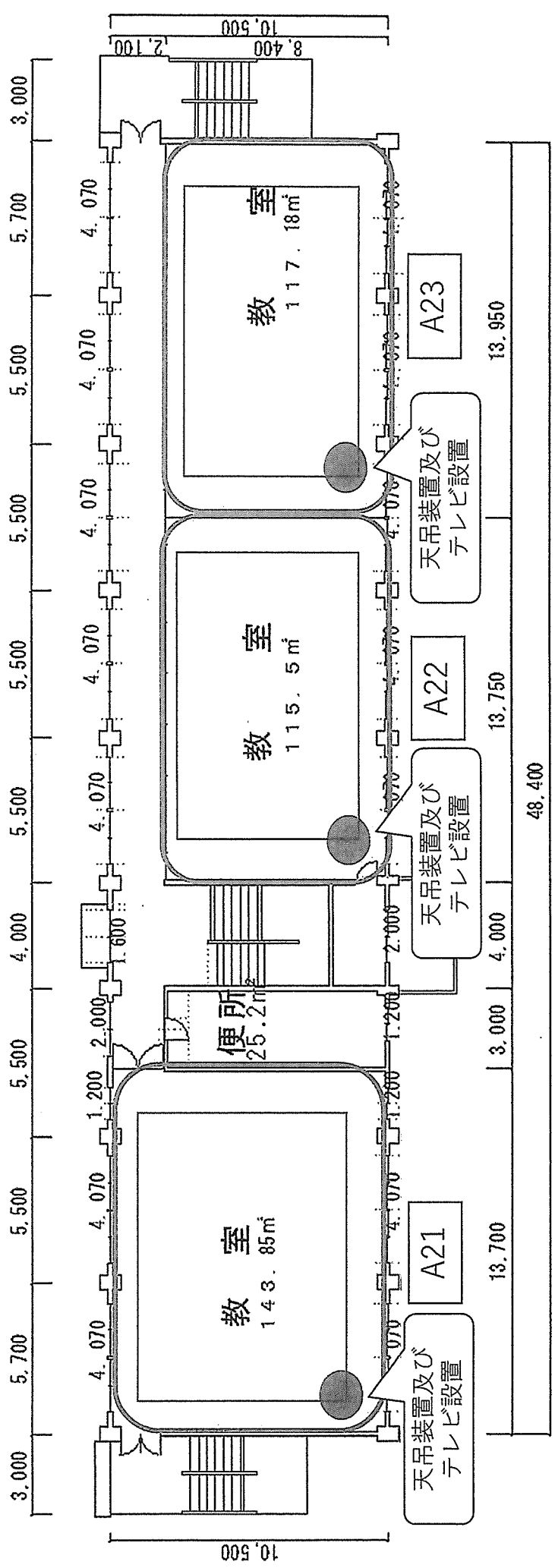
2階平面図
