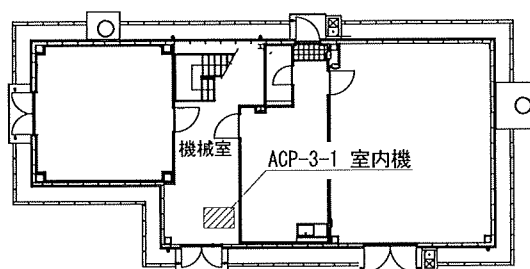
01009建物 1階平面図
