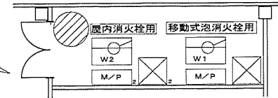
消火ポンプ室拡大図
