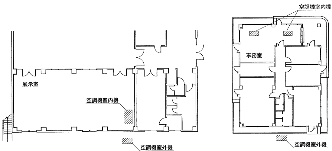
10602建物平面図
