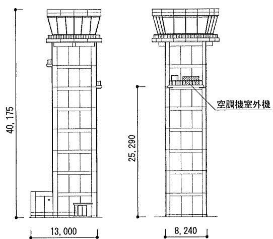
00125建物西側及び南側立面図
