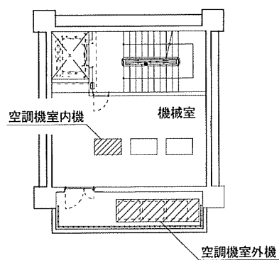
00125建物(Z7)平面図
