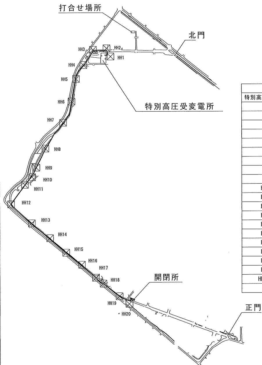
案内図 1号ケーブル配線図
