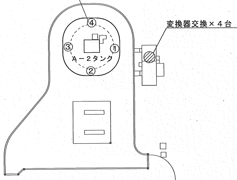
東POL漏油検知器配置図
