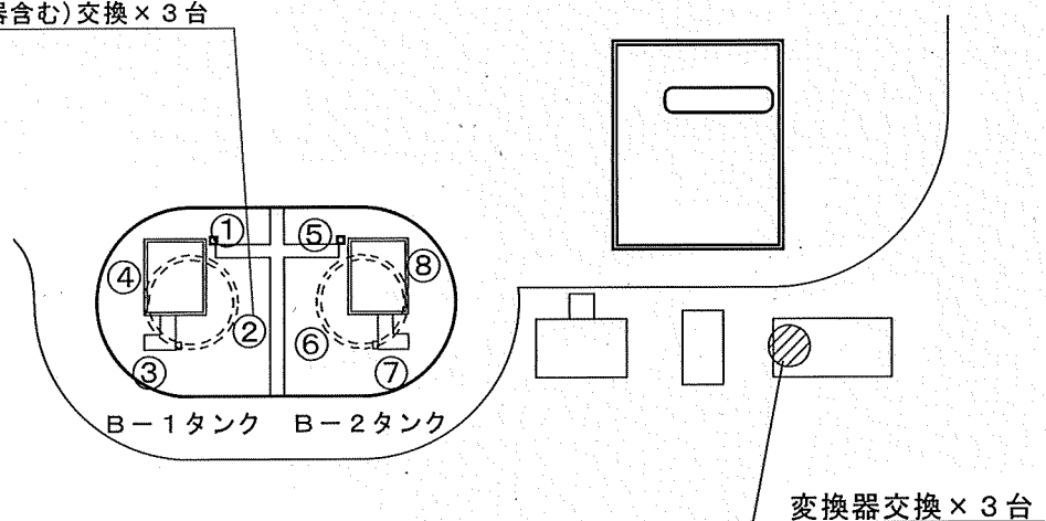
西POL漏油検知器配置図
