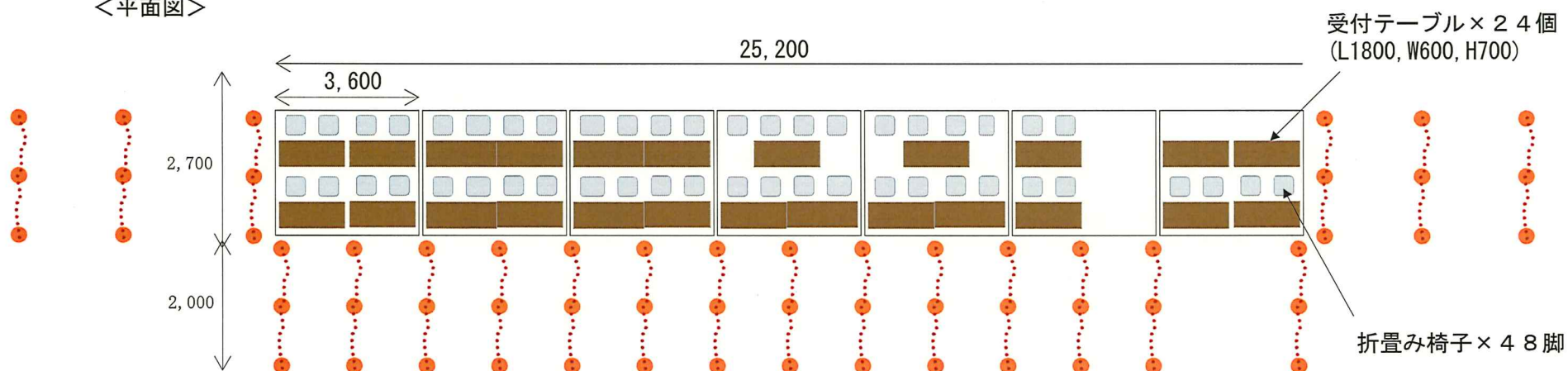
<平面図>
