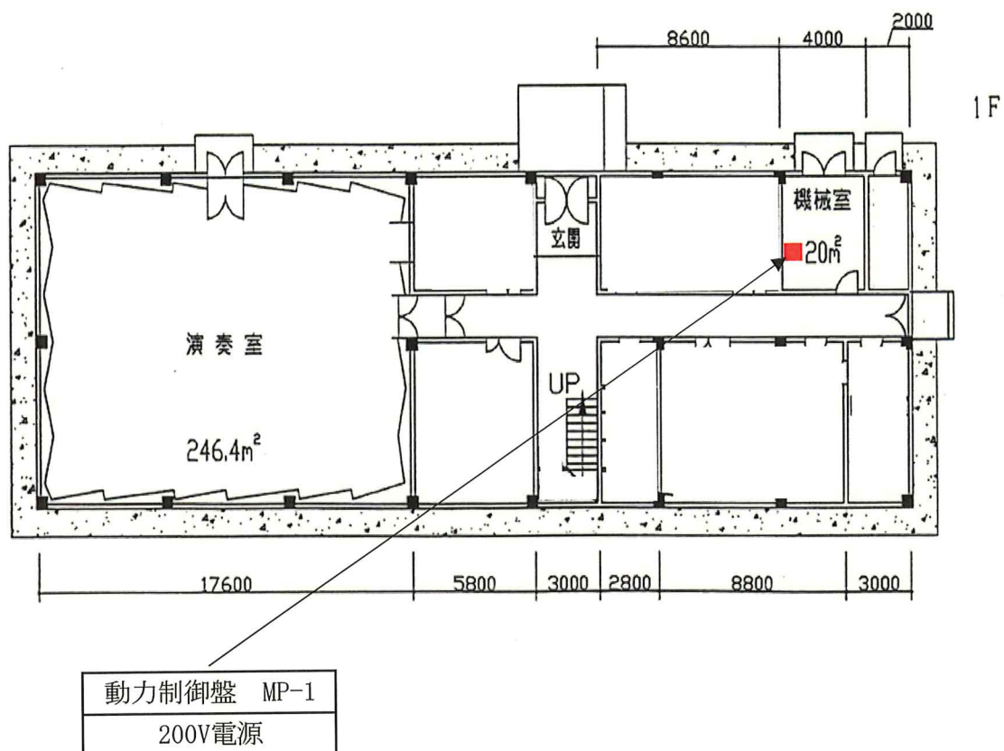
中部航空音楽隊庁舎（10548）1階平面図
