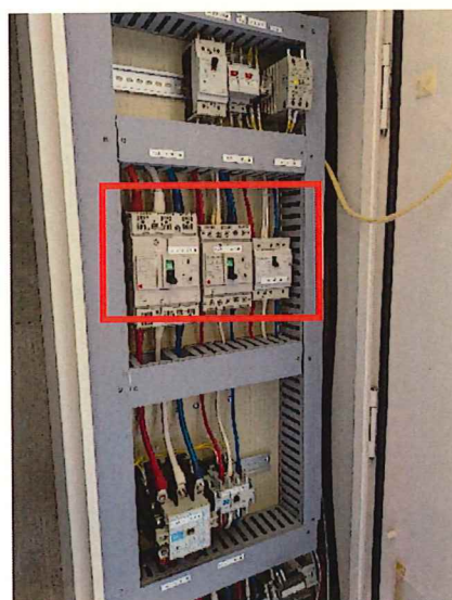
動力制御盤 内部 左から125A, 75A, 30A
