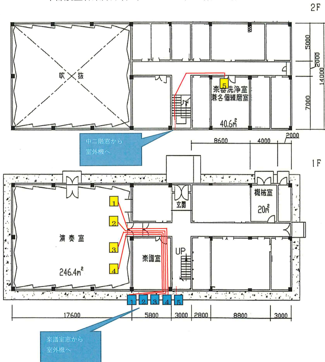
中部航空音楽隊庁舎（10548）1階・2階平面図
