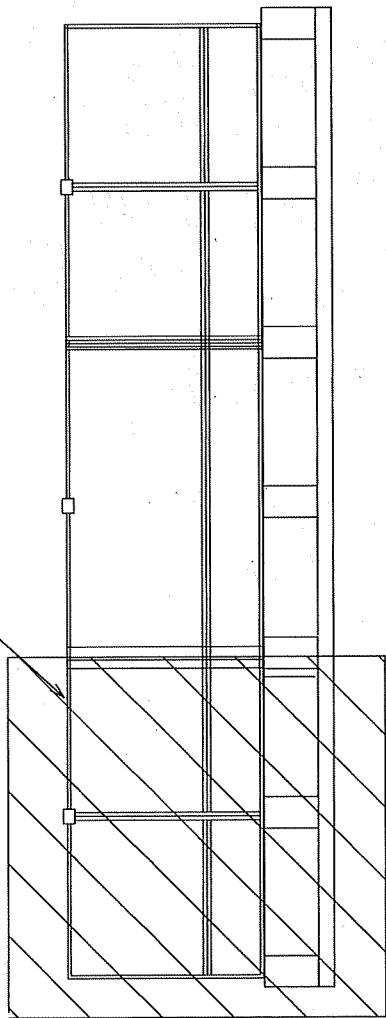
改修場所正面図
