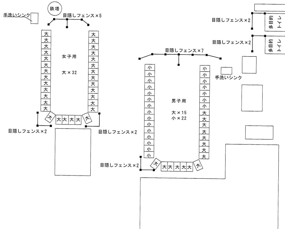
作業場所 4 設置図 (基準)
