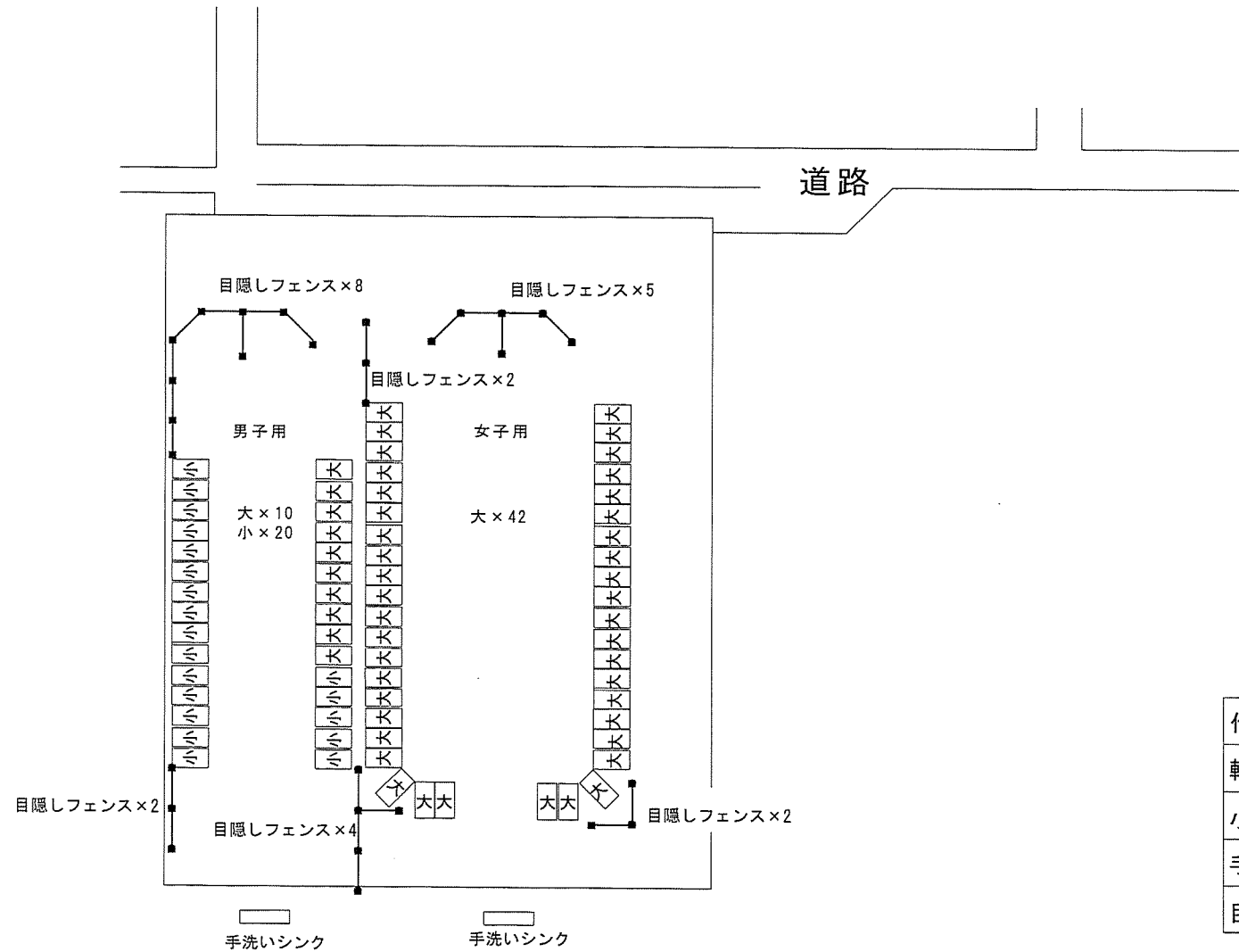
作業場所 2 設置図 (基準)
