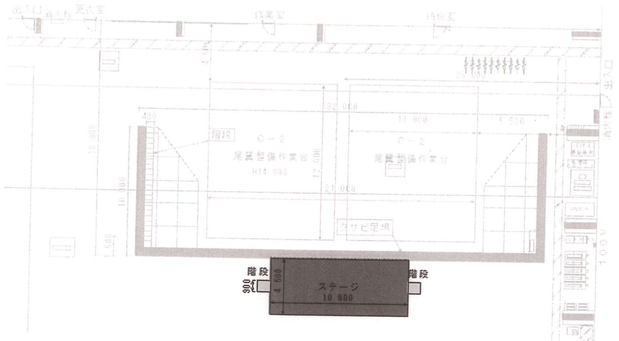
付図 ー 借上資材設置図（基準）
