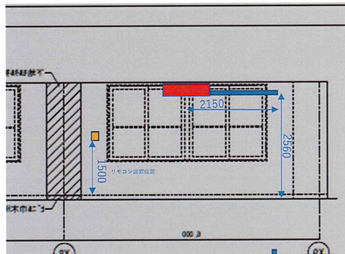
室内窓側立面図
