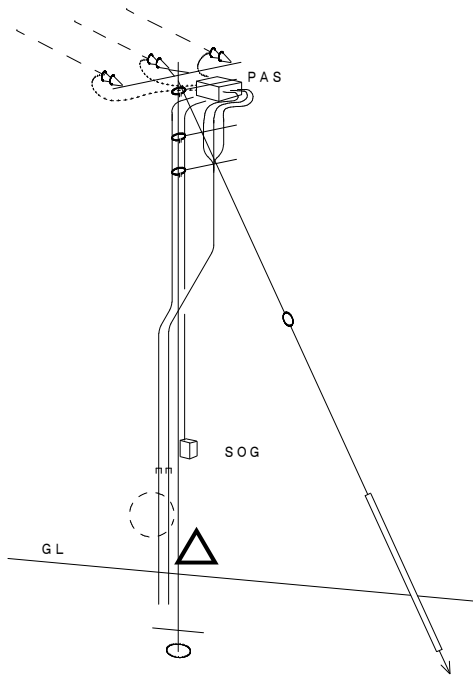
引込柱姿図
