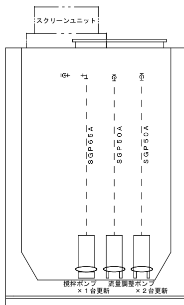
流量調整槽 断面図
