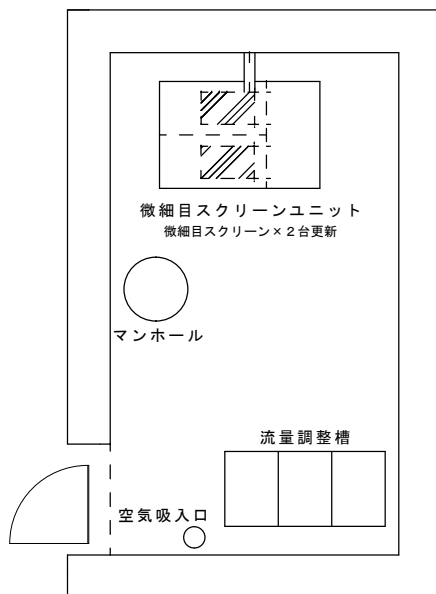
流量調整室 平面図
