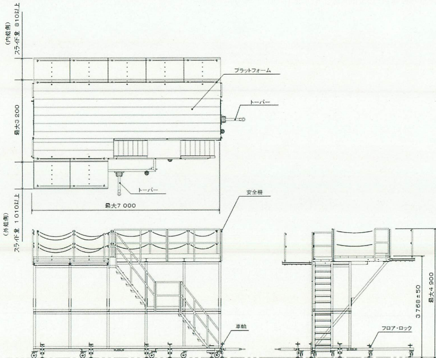
左舷バルジ台 (右舷バルジ台は対称とする。)
