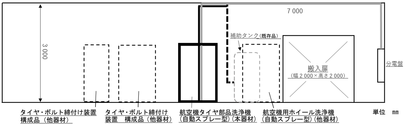
正面図
