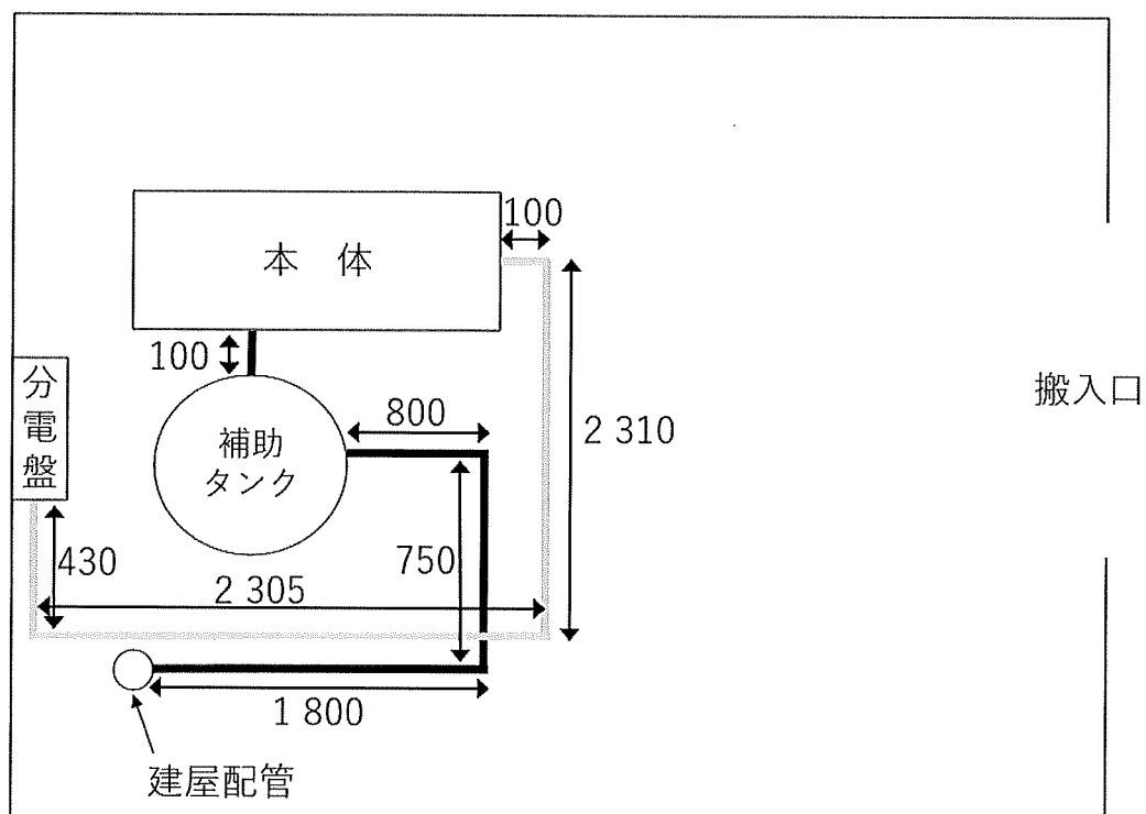
平面図
