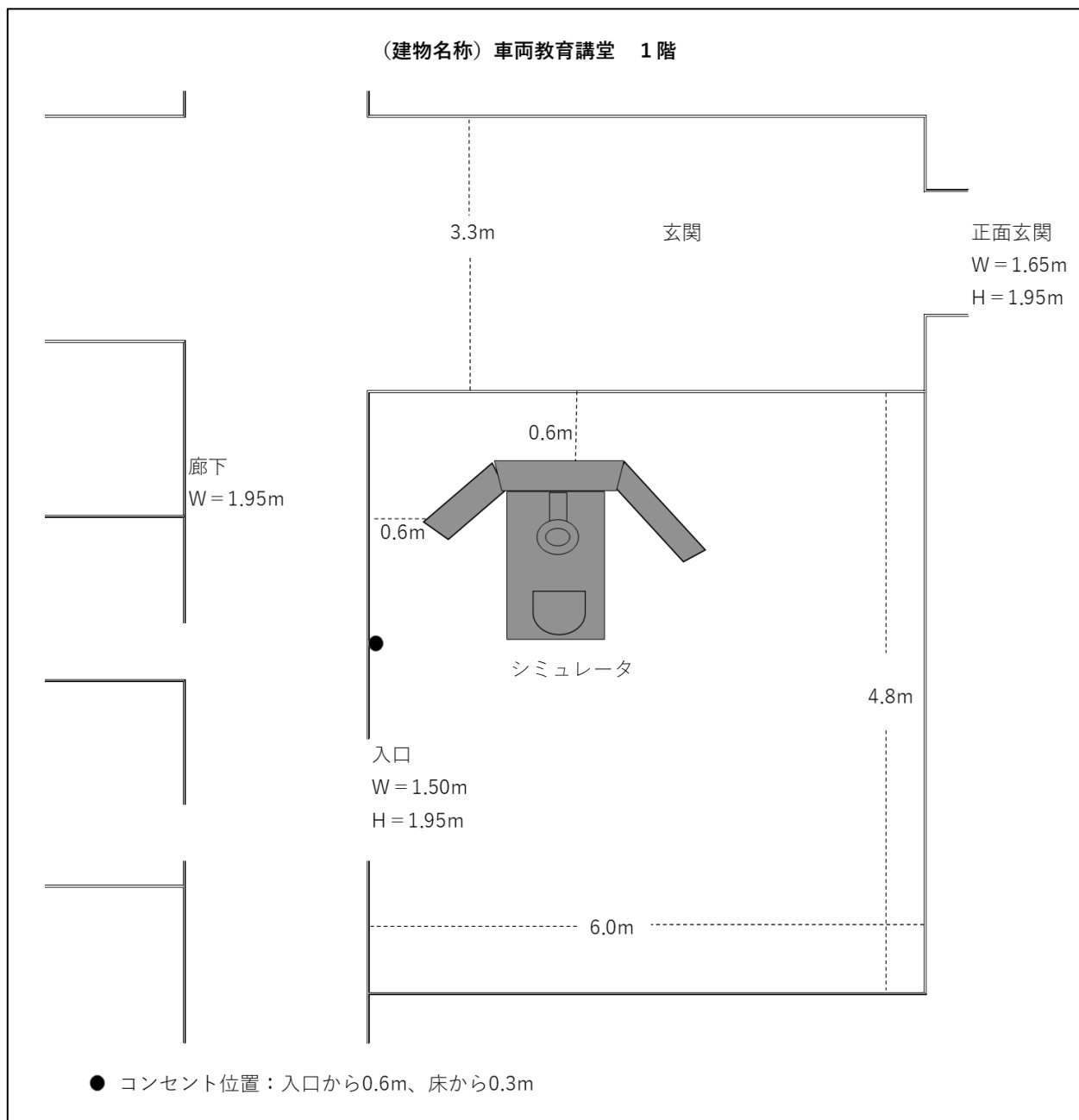
図 1－設置図
