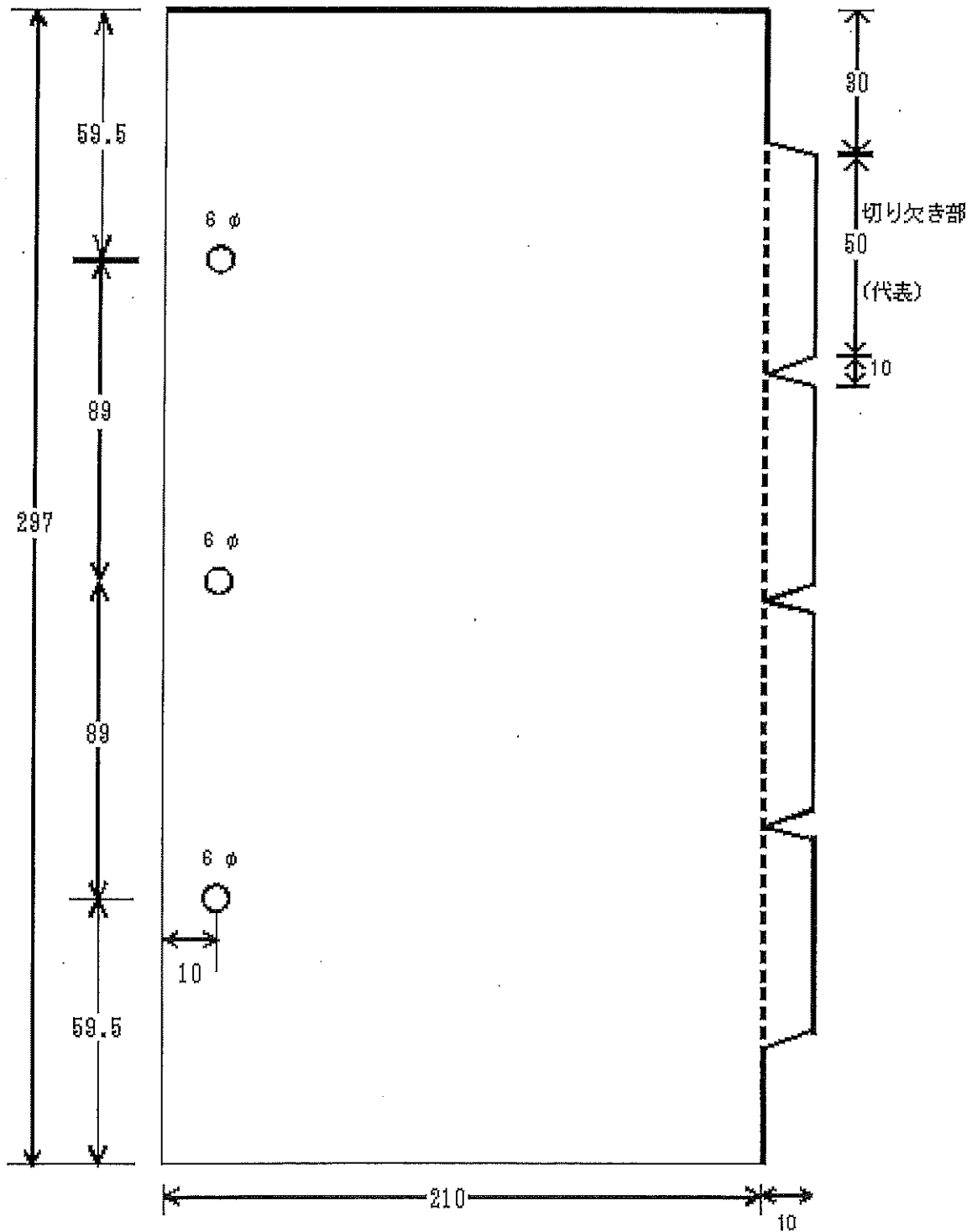
図3—仕上寸法・穴あけ位置
