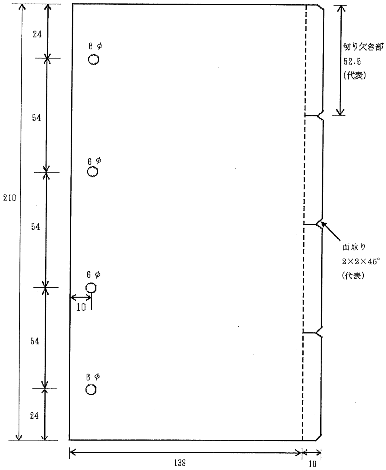
図 11—仕上寸法・穴あけ位置
