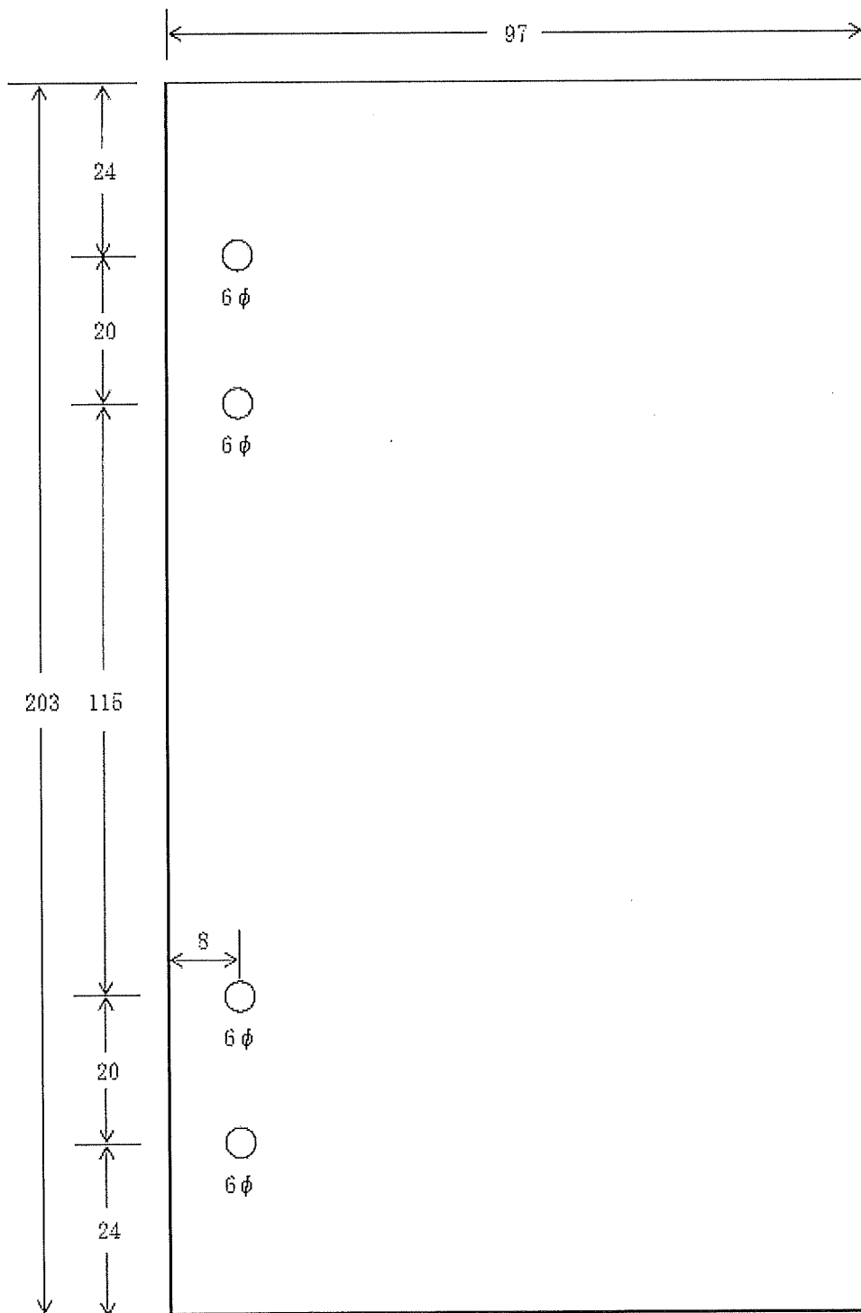
図5—仕上寸法・穴あけ位置（見出しなし）
