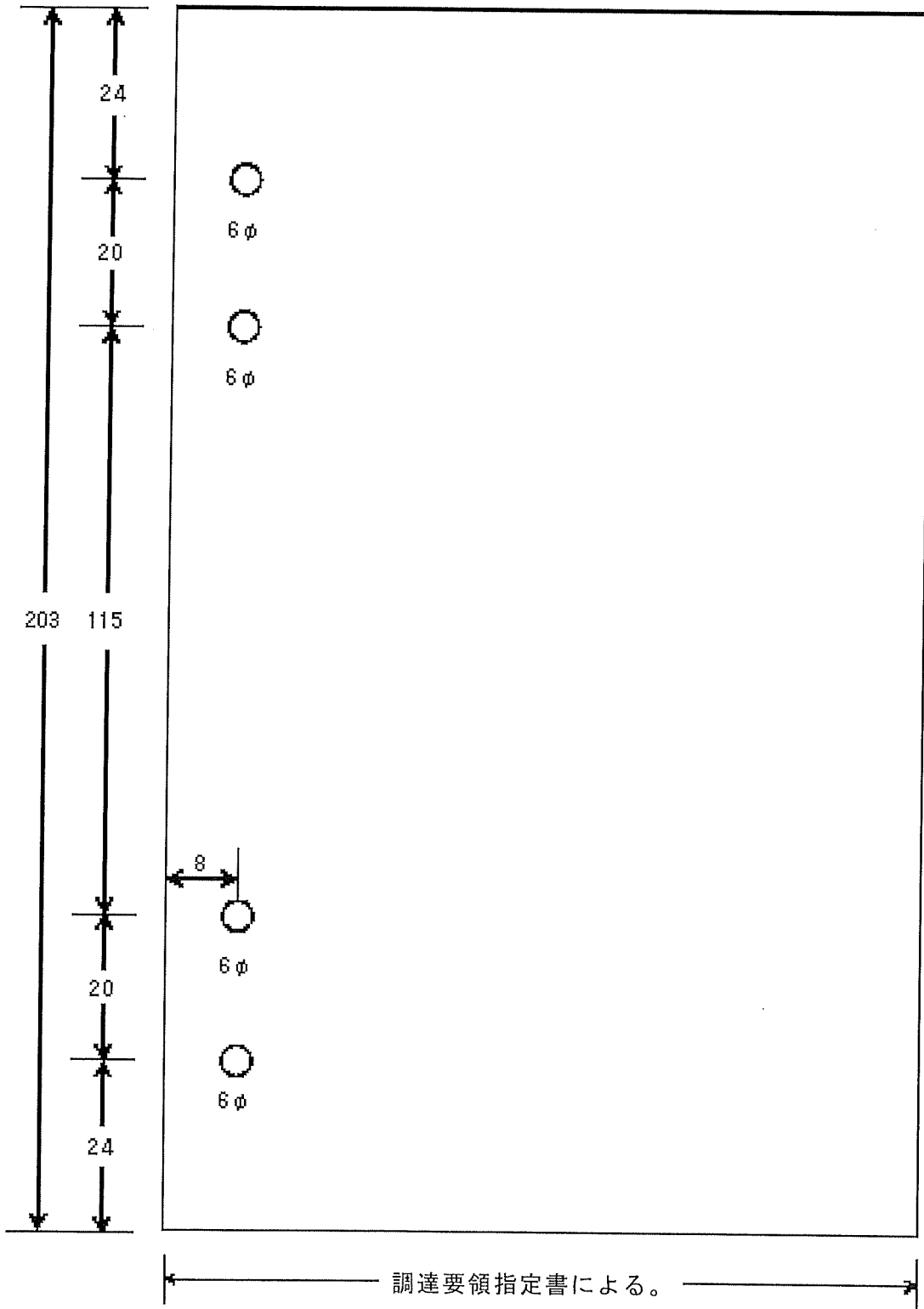
図8—仕上寸法・穴あけ位置（小型サイズ）
