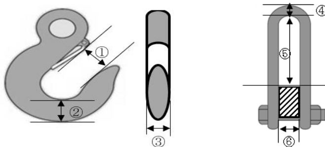
図3 - スリング吊上フック及びシャックルの諸元
