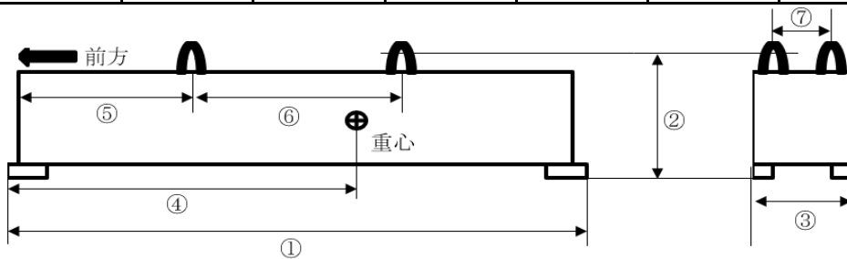
図2 - 吊上対象物の諸元
