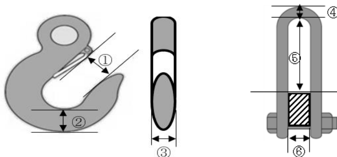
図3 - スリング吊上フック及びシャックルの諸元
