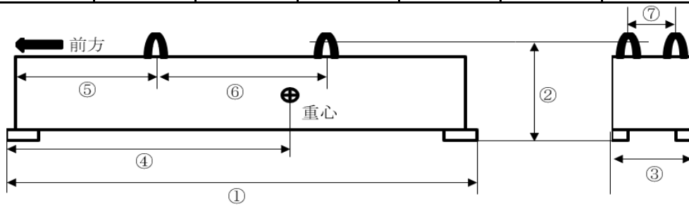
図2 - 吊上対象物の諸元
