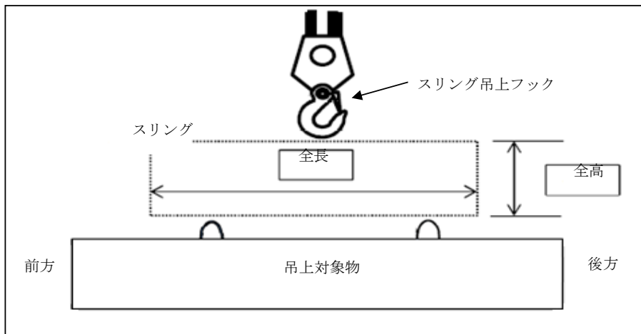
図1 - 全長及び全高等
