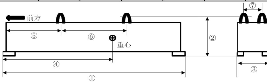
図2 - 吊上対象物の諸元
