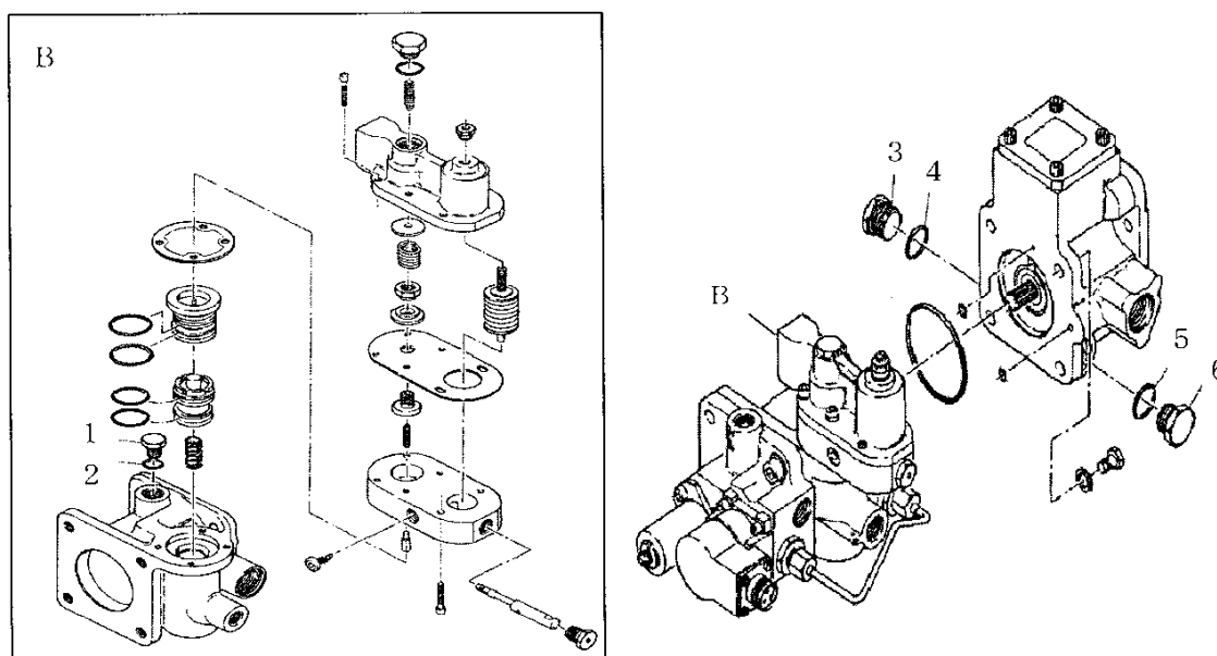
図A. 1—FUEL CONTROL外観
