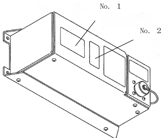
図A. 1-CONTROLLER外観
