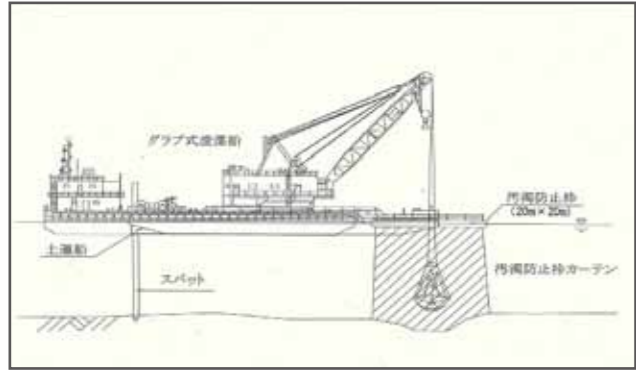
しゅんせつ状況図(側面図)
