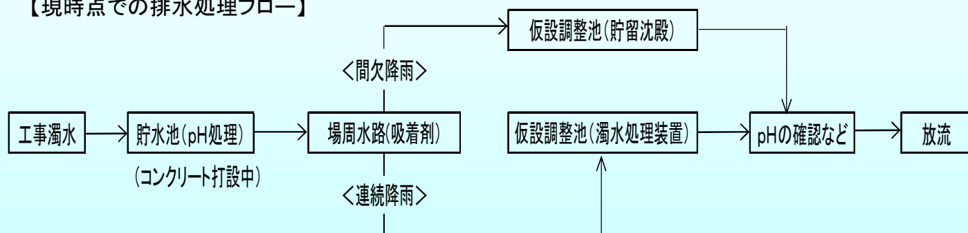
【現時点での排水処理フロー】
