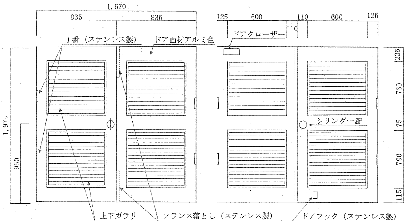
3階大会議室入口ドア姿図 (通路側) 1 : X
