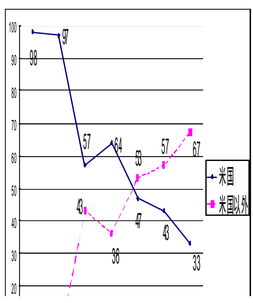
船舶用燃料消費量の比率の推移
