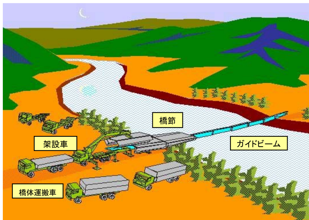
運用構想図
