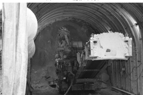
坑道式陣地の構築 (第302坑道中隊)
