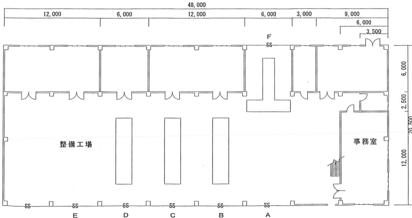
1階平面図
