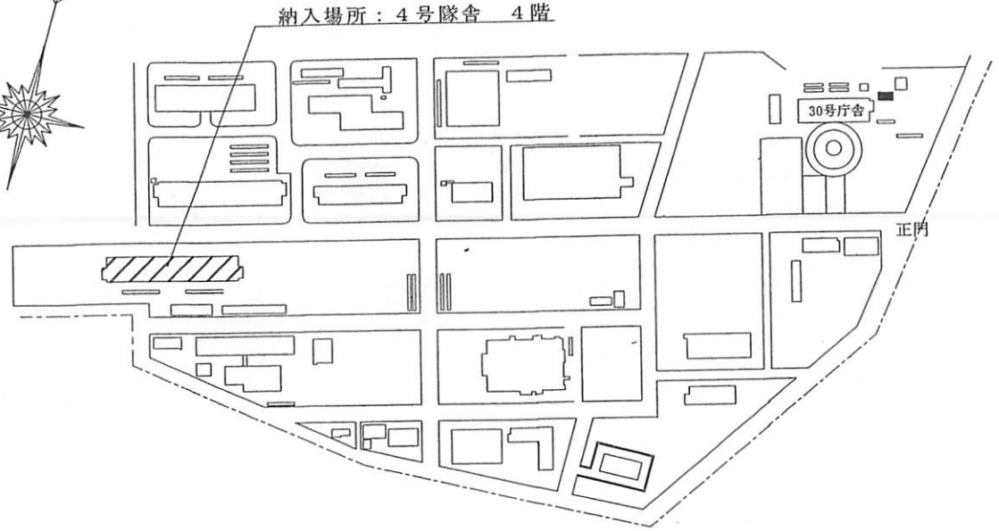
配置図 S=1/7000
