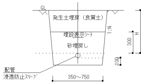
一般部標準図 S=1/30
