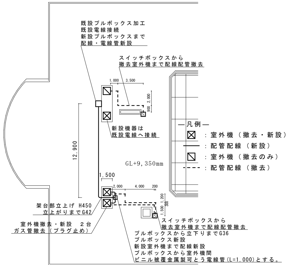
R階平面詳細図 S=1/300
