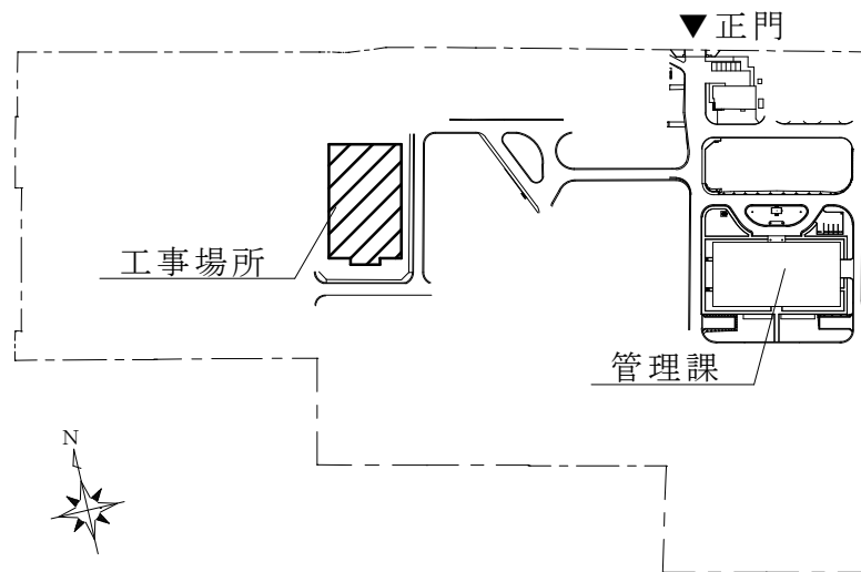
配置図 S=1/X
