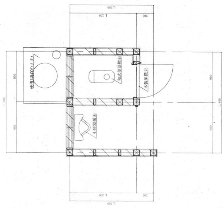
補修前平面図 S=1:30
