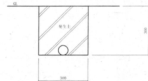
標準断面図 S=1:10
