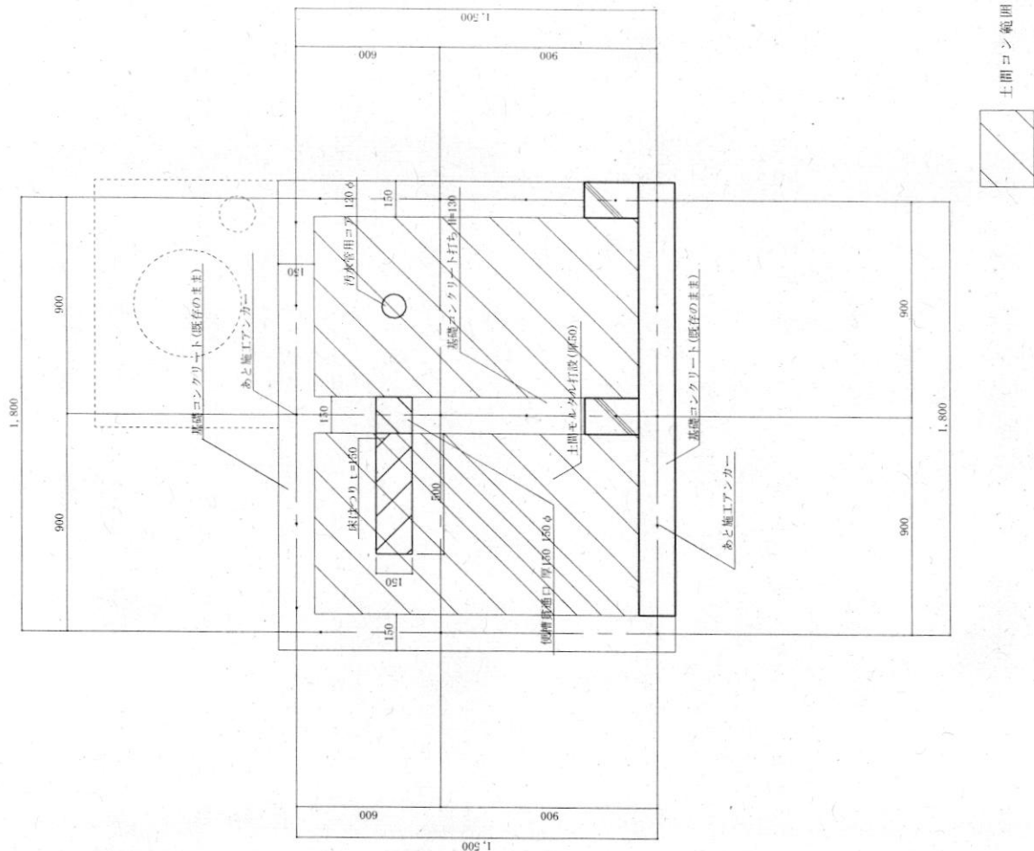
補修後基礎伏図 S=1:20
