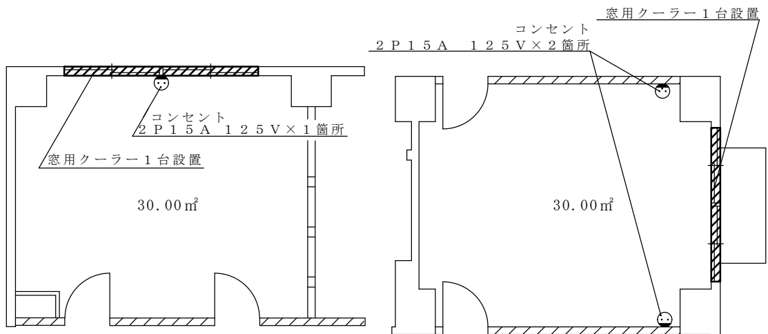
居室標準平面図 S=1/Non
