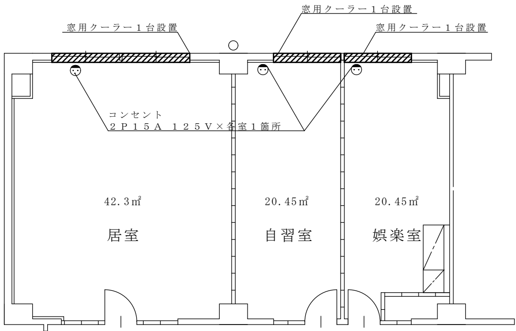
50号建物設置標準図 S=1/X
