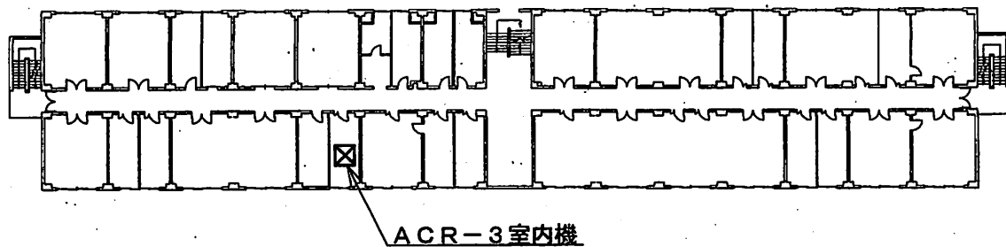
1号建物 2階平面図 S=1/X
