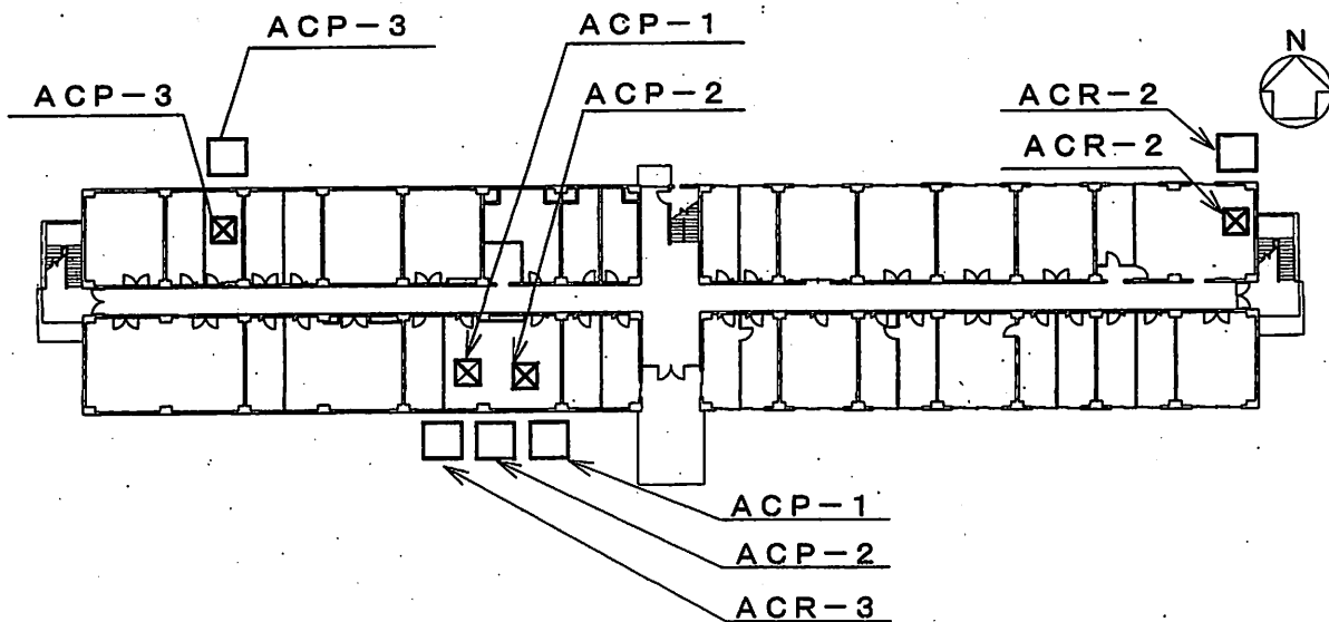
1号建物 1階平面図 S=1/X
