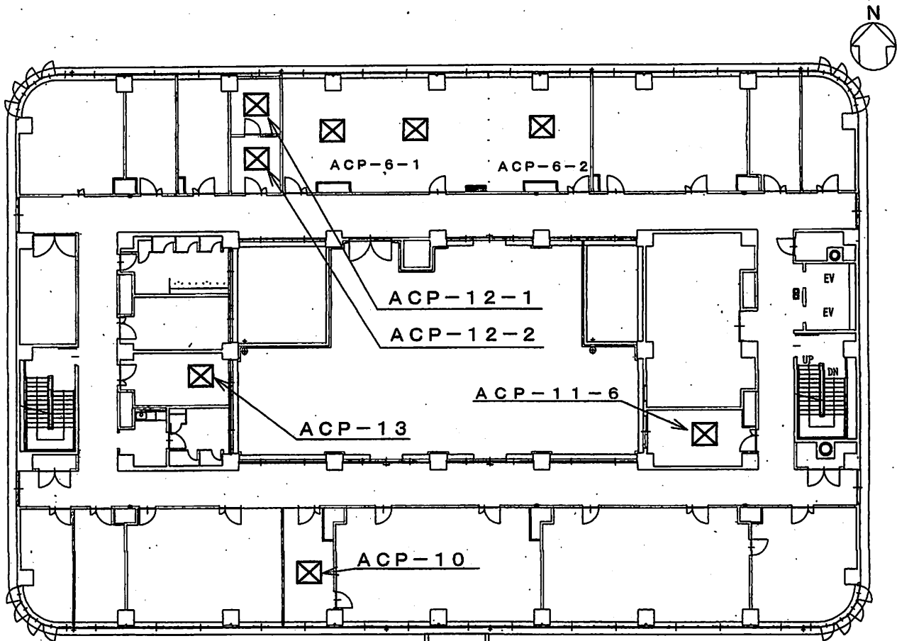
13号建物 3階平面図 S=1/X
