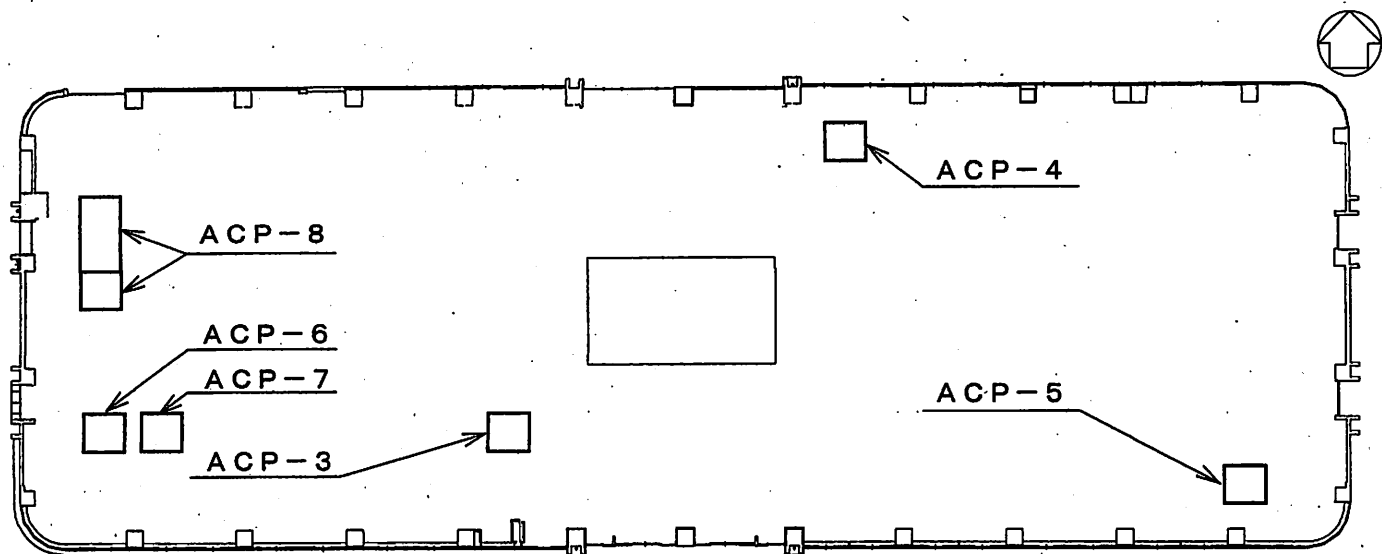
14号建物 屋上平面図 S=1/X
