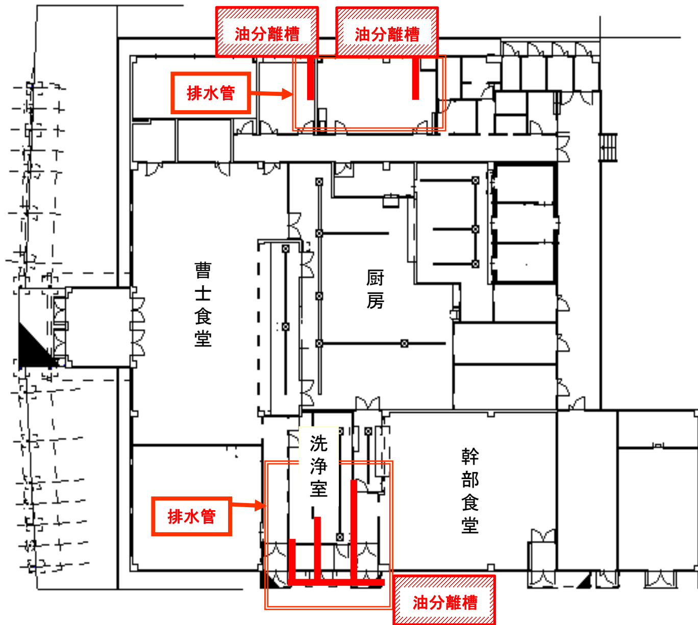
图 1 — 松戸駐屯地隊員食堂平面図
