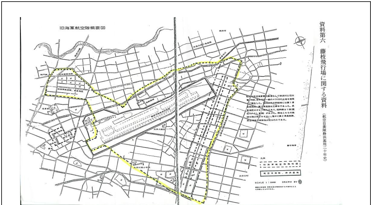
藤枝海軍航空基地全体図
