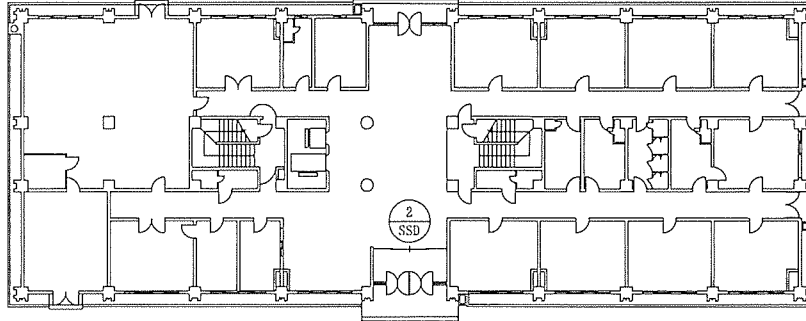
#218 平面図 S=1/500
