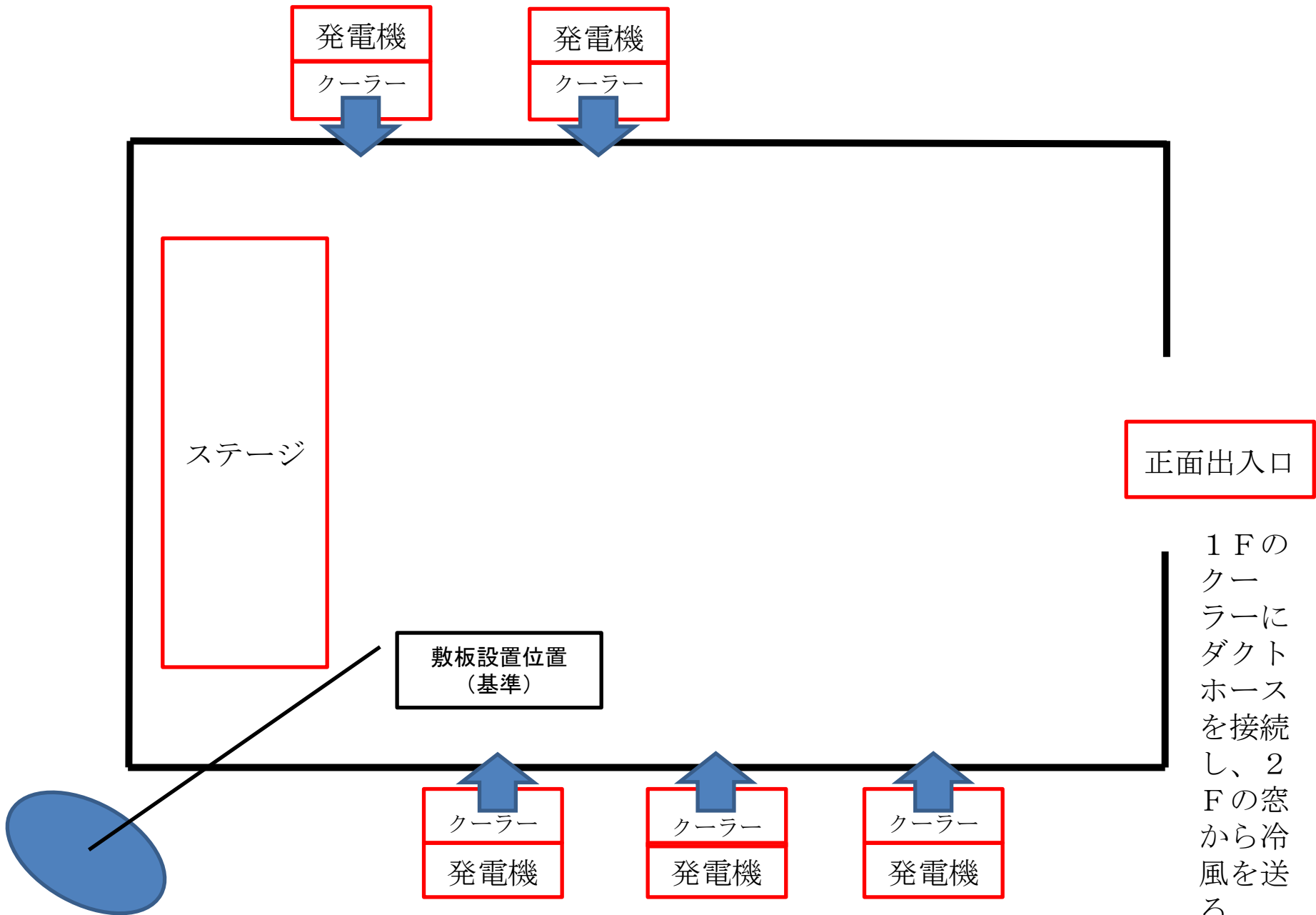
付図ー1 基地体育館屋外周辺設置レイアウト (基準)
