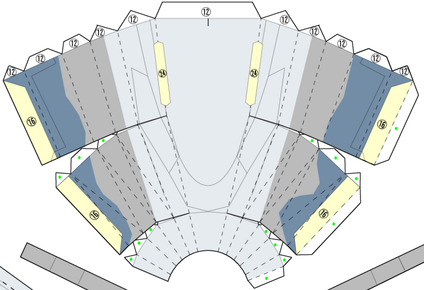
11 機体後部2
