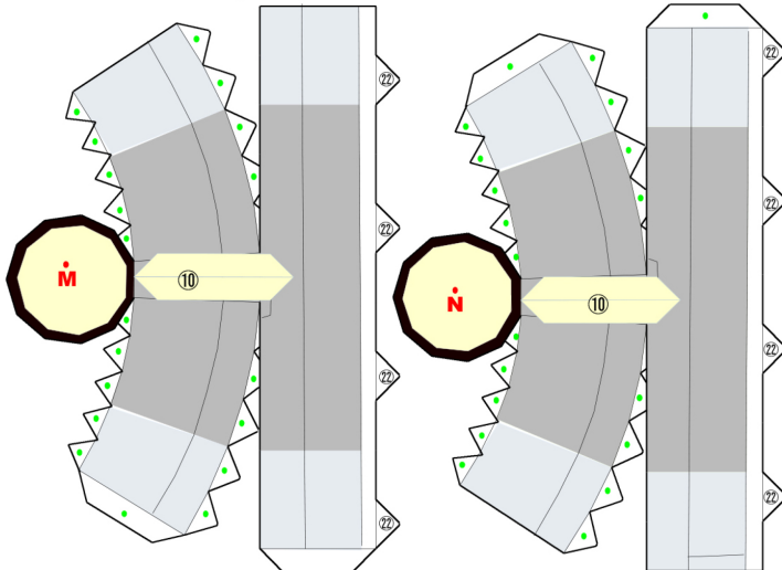
20 エンジン前部1
