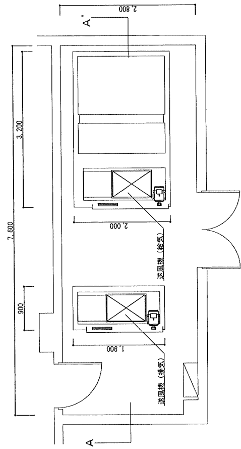
#91 食厨 機械室 平面図 S=NON
