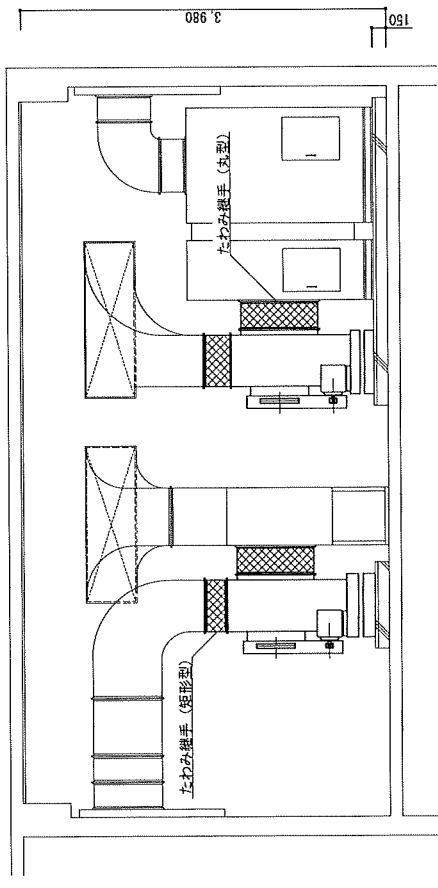
#91 食厨 機械室 A-A' 断面図 S=NON
