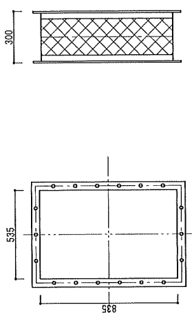
たわみ継手(矩形型)詳細図 1/30
