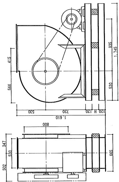
IFA 5SRM2型片吸込マルチファン 詳細図 S=NON
