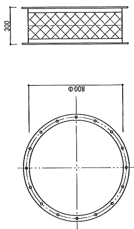
たわみ継手(丸形)詳細図 1/30
